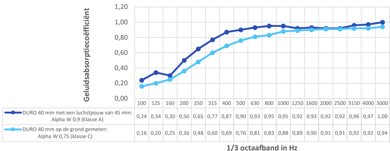
Geluidsabsorptie in functie van de frequentie
